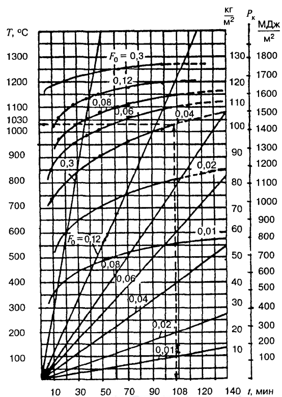
Рис. 5. Номограмма для определения максимальной среднеобъемной температуры и времени ее достижения при ПРВ
