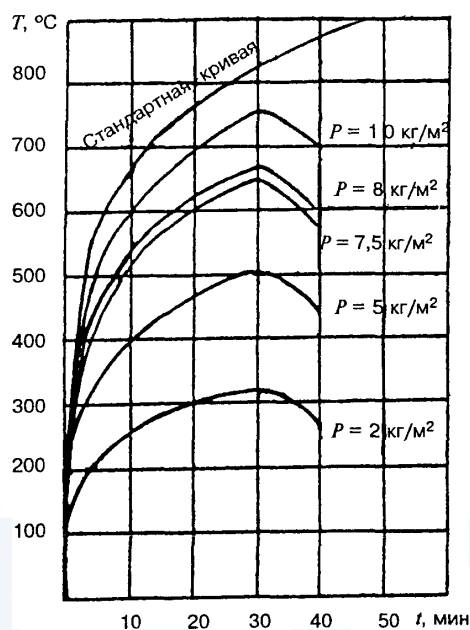
Рис. 4. Температурные режимы ПРН
