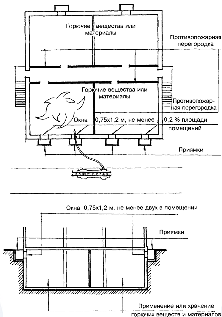
Рис. 2. Устройство окон с прямыми в подвальных этажах
