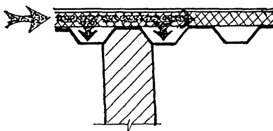
Рис. 1. Варианты возможного распространения пожара
