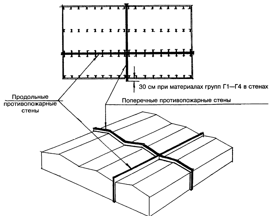
Рис. 4. Разделение зданий на пожарные отсеки противопожарными стенами
