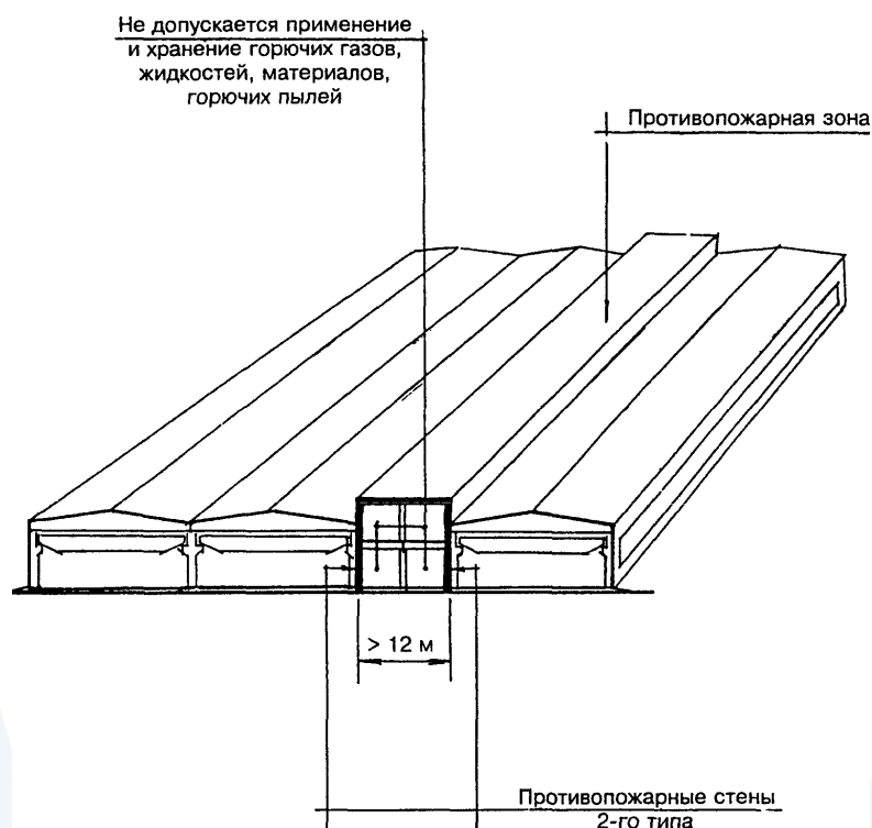
Рис. 9. Противопожарная зона
