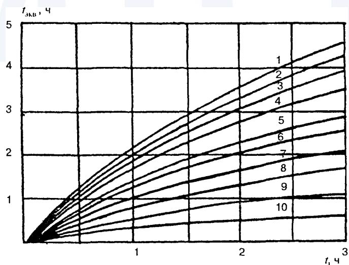
Рис. 6. Зависимость эквивалентной продолжительности пожара для железобетонных плит перекрытия от времени пожара для ПРВ
